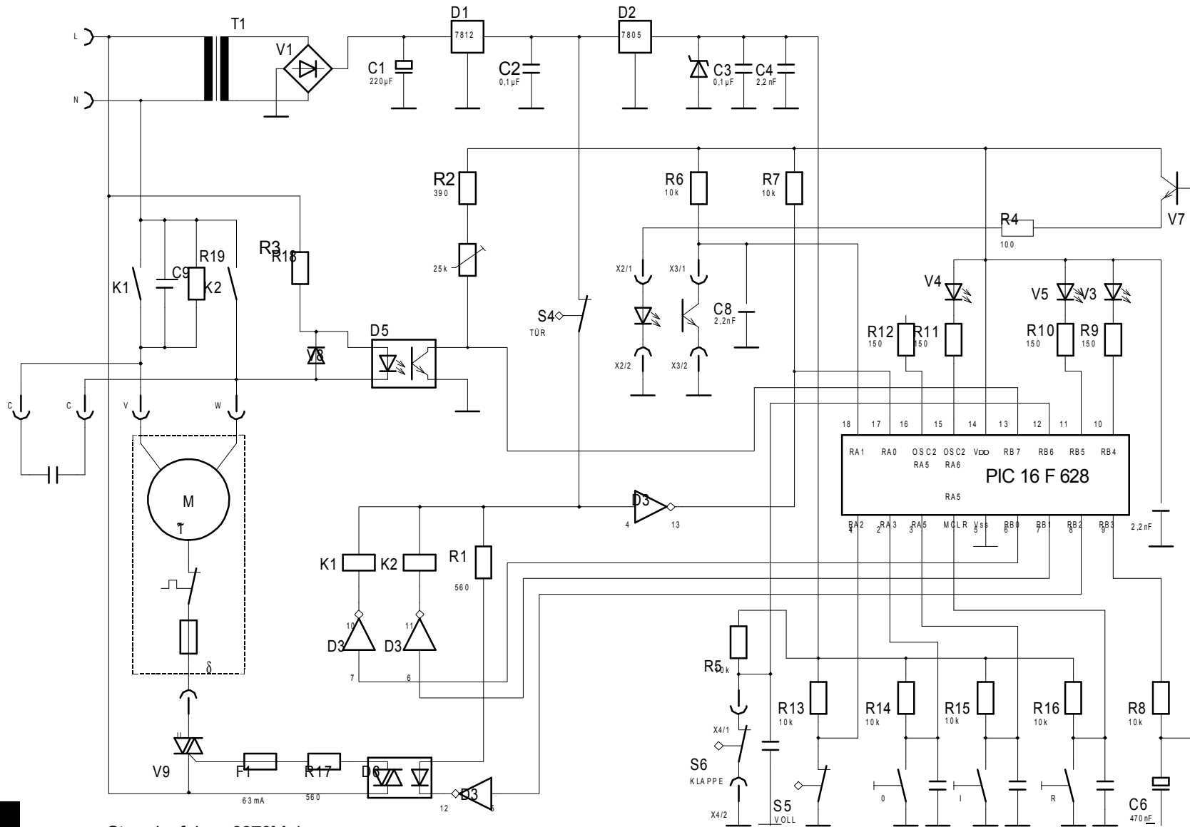
Stromlaufplan 3870M-1 schema de circuit électrique 3870M-1 wiring diagram 3870M-1
