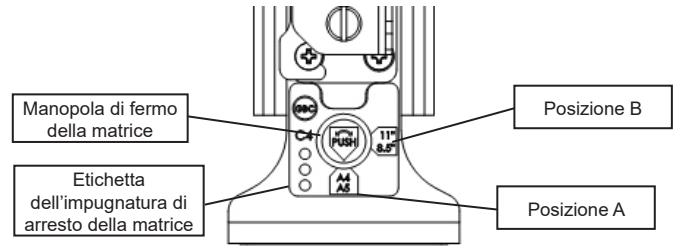
Figura 8.7 Posizione di fermo della matrice a spirale
