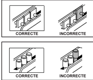
Figure 8.5 Ajout de poinçons
