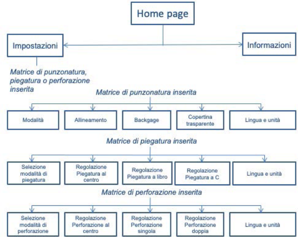
Descrizione del pannello LCD
