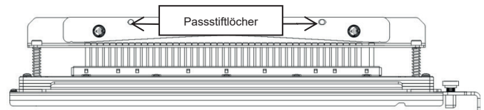
Abbildung 8.4 Druckleiste einbauen
