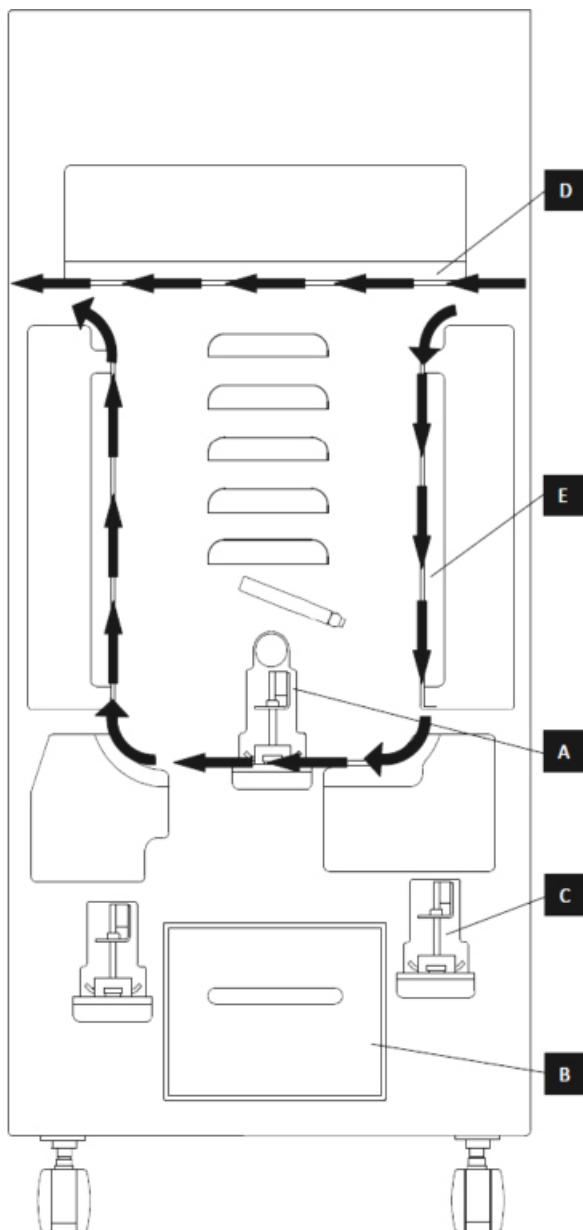
Papierführung und interaktive Bedienelemente des StreamPunch Plus
