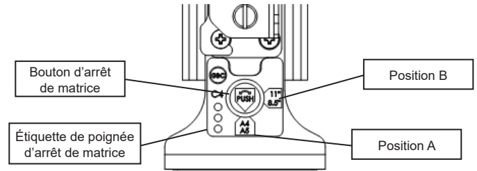
Figure 8.7 Position d'arrêt des matrices à bobine
