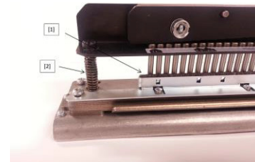
Figura 8.8 Lubricación
