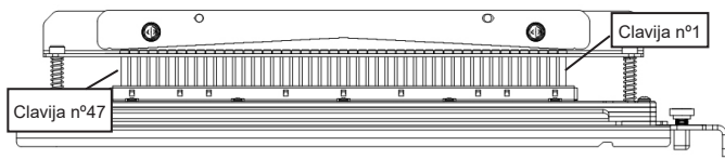
Figura 8.1 Numeración de clavijas de juego de troqueles para espiral
