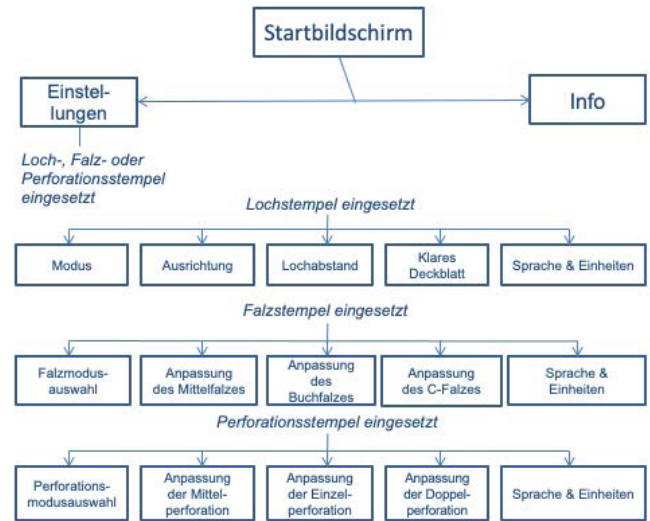
Übersicht LCD-Anzeige
