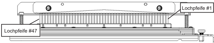
Abbildung 8.1 Nummerierung der Lochpfeifen eines Spiral-Lochstempels
