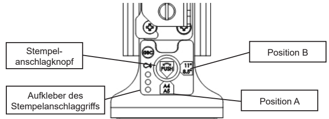
Abbildung 8.7 Spiral-Lochstempelanschlagsposition
