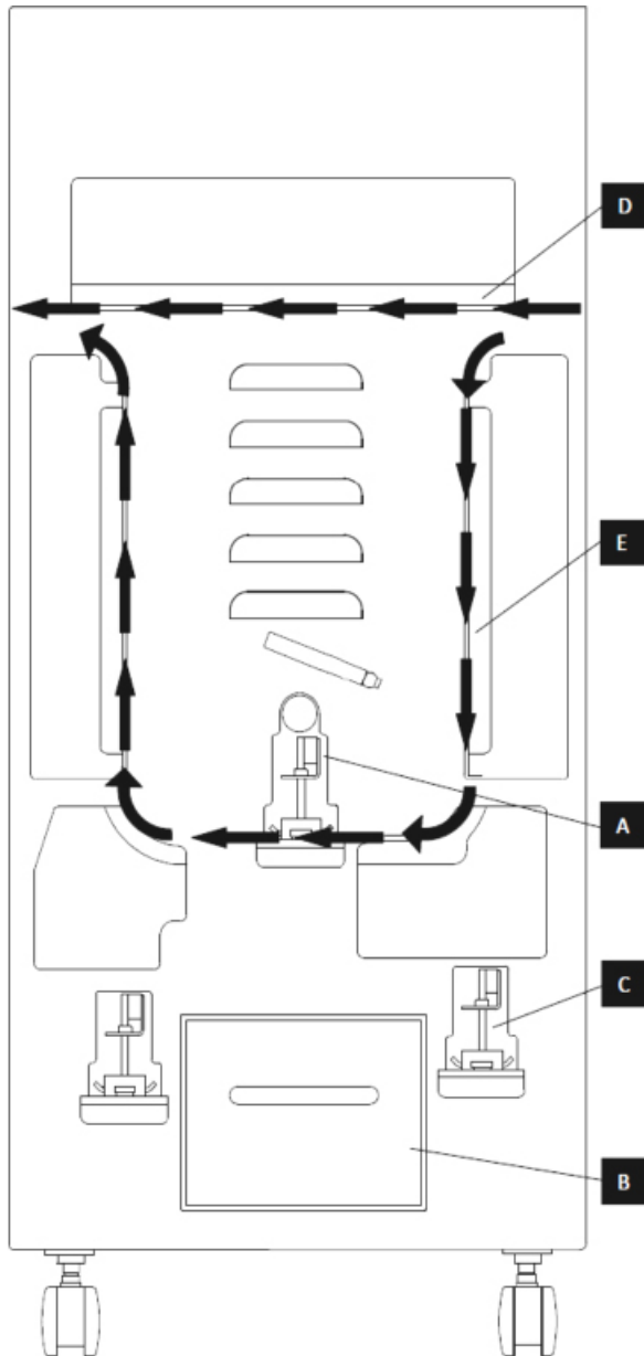
Flujo del papel y secciones Interactivas de Usuario de StreamPunch Plus
